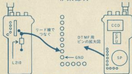
C500 クロスバンドレピータ改造ポイント
